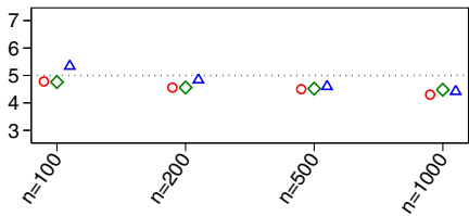
Minimisation
